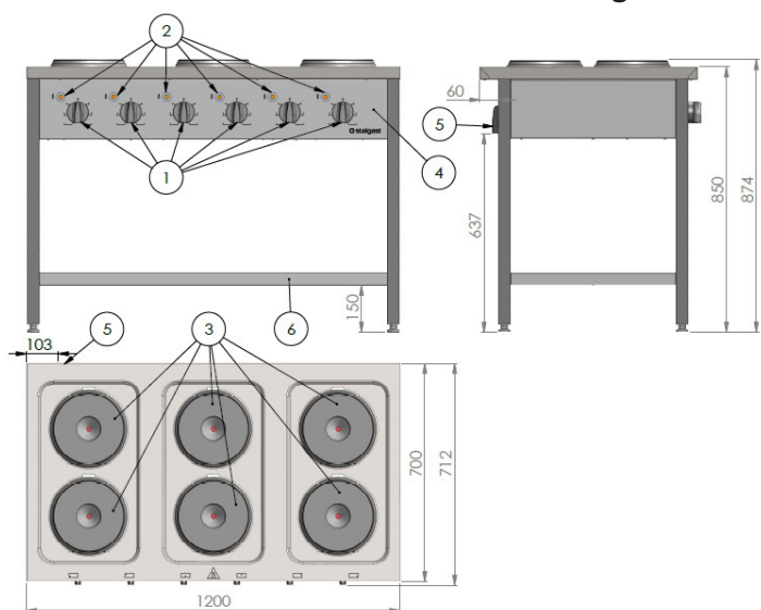
Abb. 3 Abmessungen eines Elektro-Herds 700 6x2,6 kW
