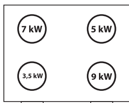
Obrázok 6. Umiestnenie horákov na sporáku so štyrmi horákmi (schematicky)
