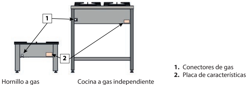
Figura 15. Vista trasera del dispositivo.
